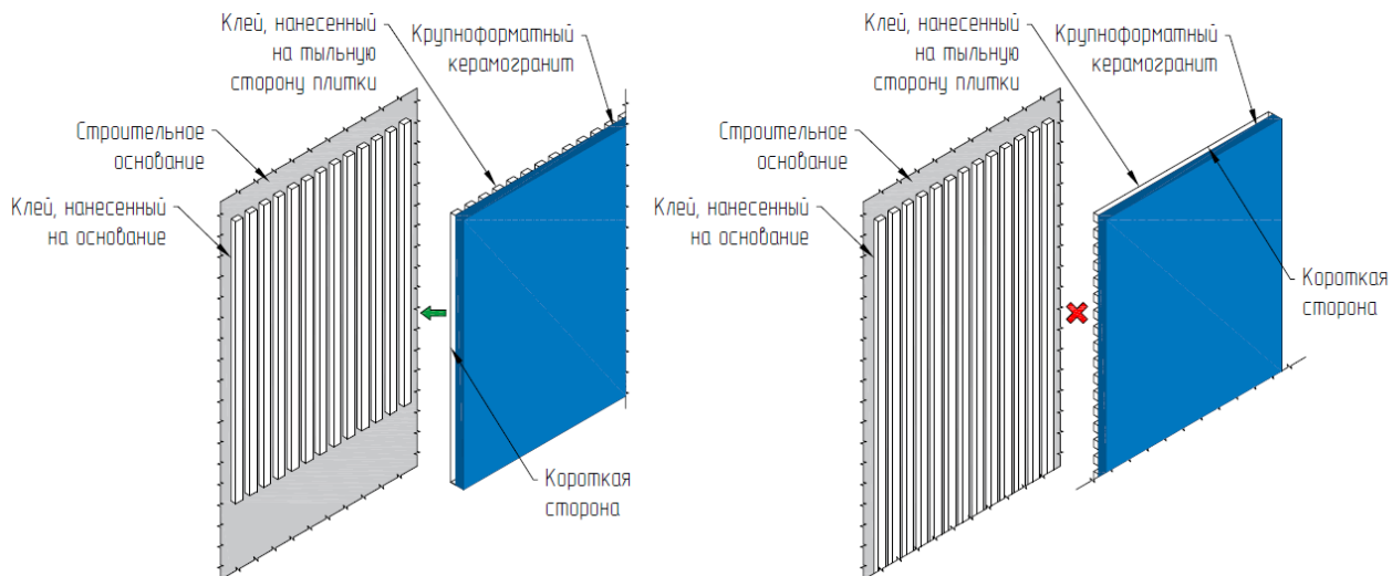
Рис. 35. Клей следует наносить в одном направлении на основание и на плитку
