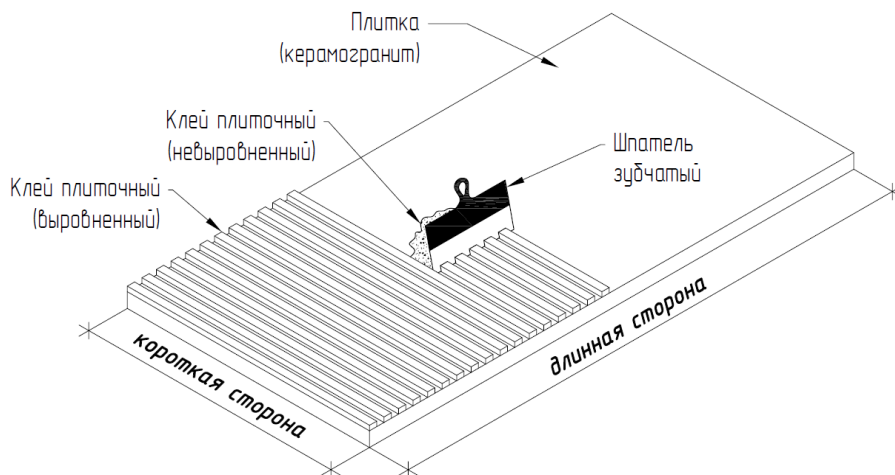
Рис. 34. Нанесение плиточного клея на плитку
