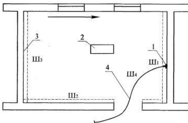
Рис. 27. Схема организации рабочего места звена № 1
